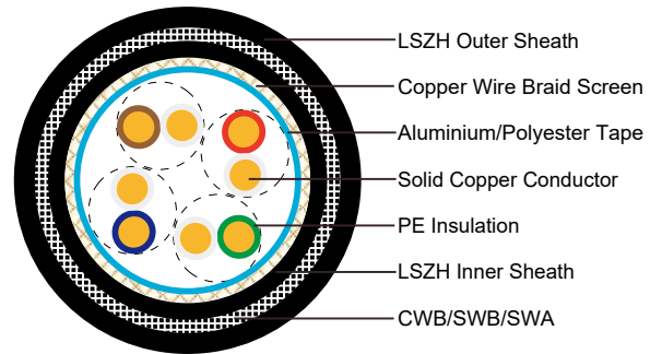
SF/UTP CAT5E
