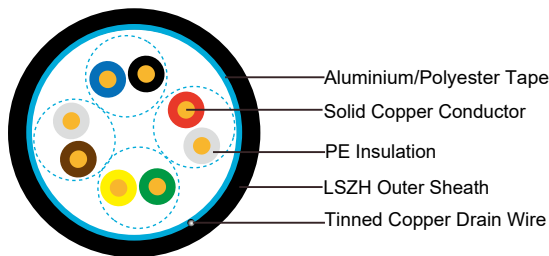
F/UTP CAT5E
